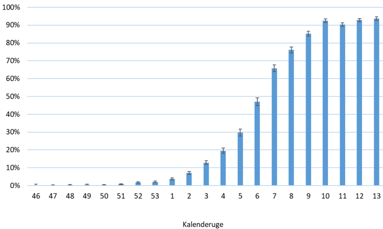
Figur 2. Andel af sekventerede prøver med B.1.1.7 med 95% konfidensintervaller, uge 46 2020 til uge 13 2021.
